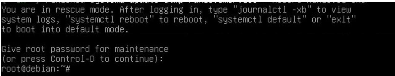
aktivierter Wiederherstellungsmodus
