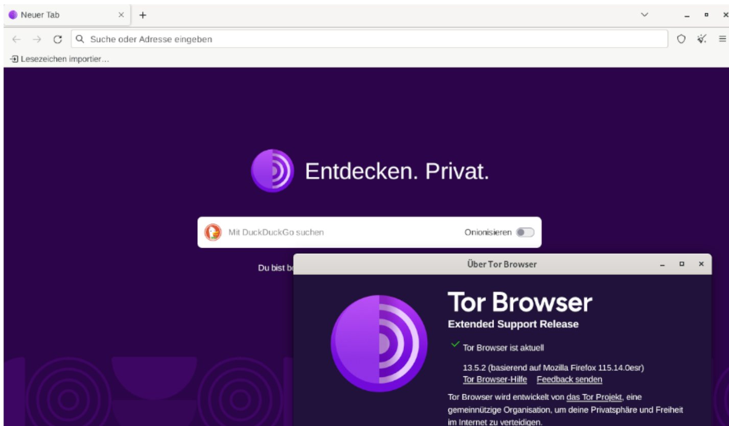
Tor Browser
