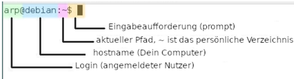
Terminal Präsentation
